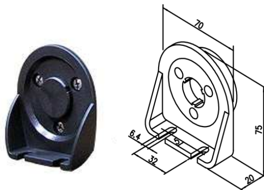
L 型邊蓋
